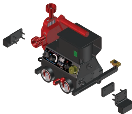
BLO-0466-48-01-00-0 Magnetni blokovi (zadnji) sa povećanom snagom M6x25
