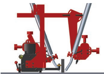
PDT-0466-40-00-00-0 Postolje za 2 gorionika
